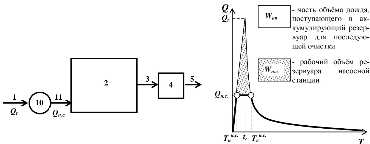
Рис. 3. Схема 1 перекачки полного объема незарегулированного дождевого стока. 10 – насосная станция 11 – напорный трубопровод перекачки стока в аккумулирующий резервуар.
